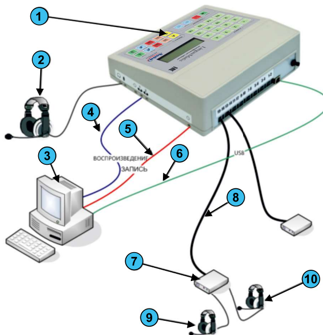
Рис.6 Схема подключения
